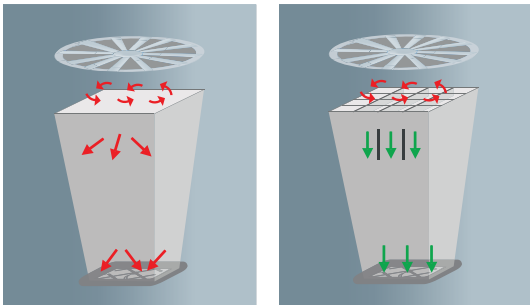
Principio di funzionamento del raddrizzatore di flusso
